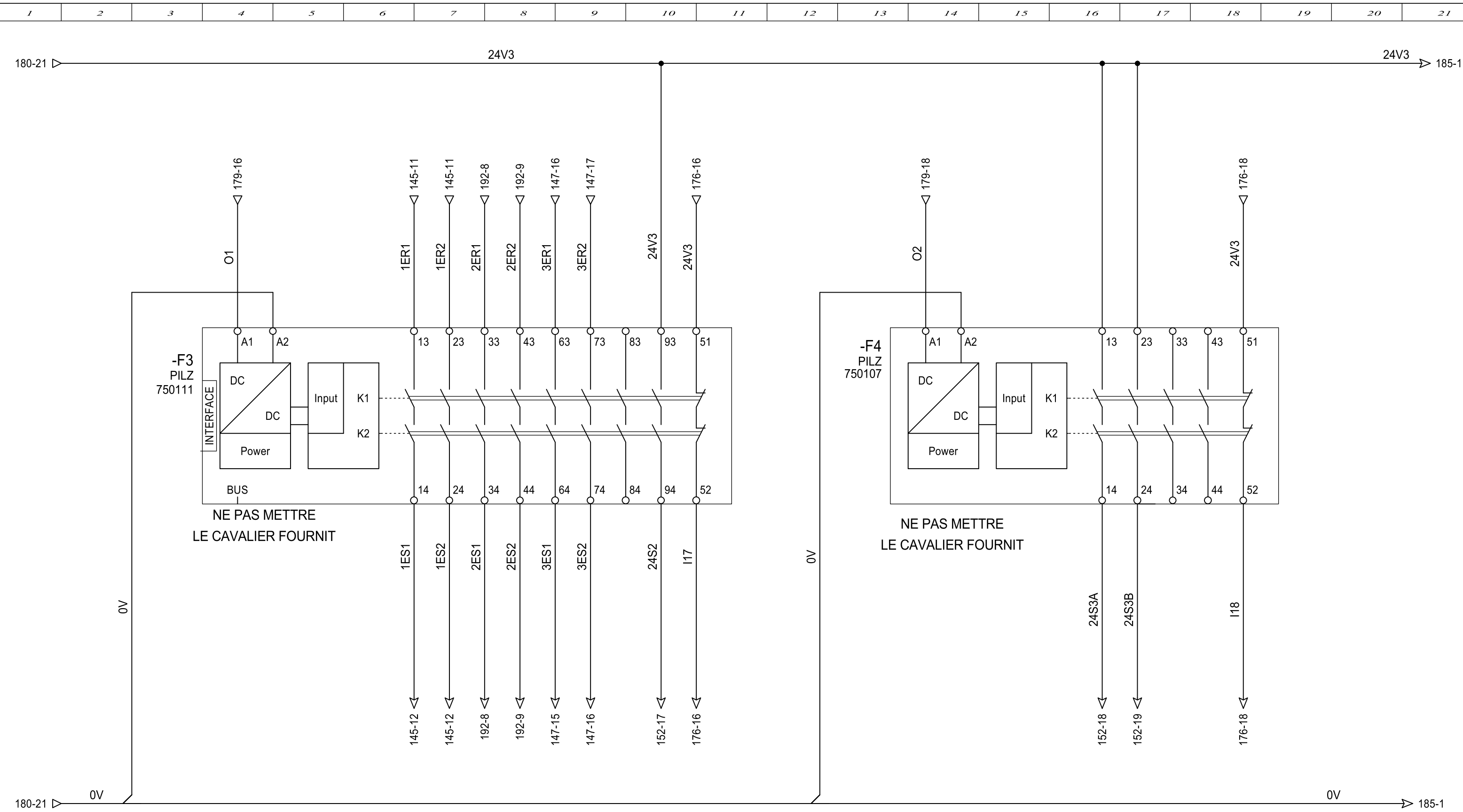
RELAIS DE SÉCURITÉ ARU + ENCEINTE
