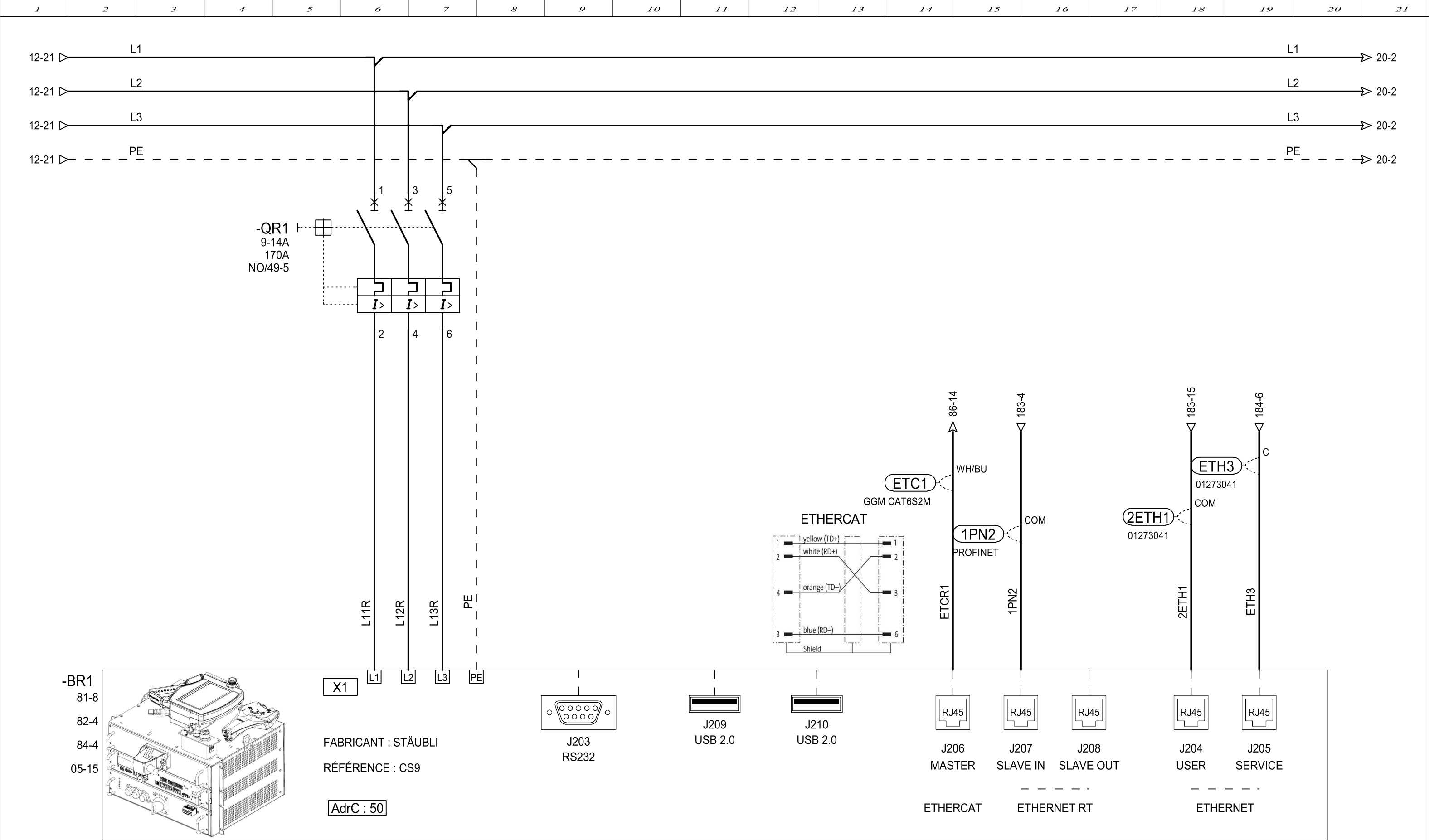
BAIE ROBOT 1 2 kVA
